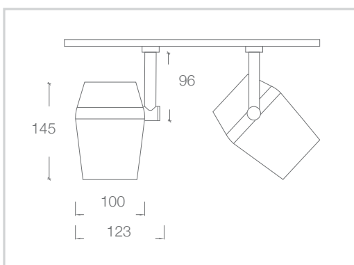
Black baffle IC66.BF
