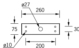
Mounting detail Instructions de montage Asennusohje
